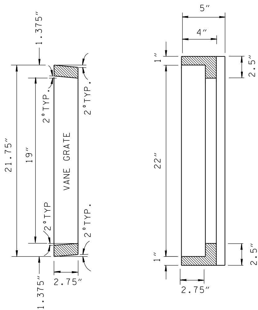
SECTION D-D
